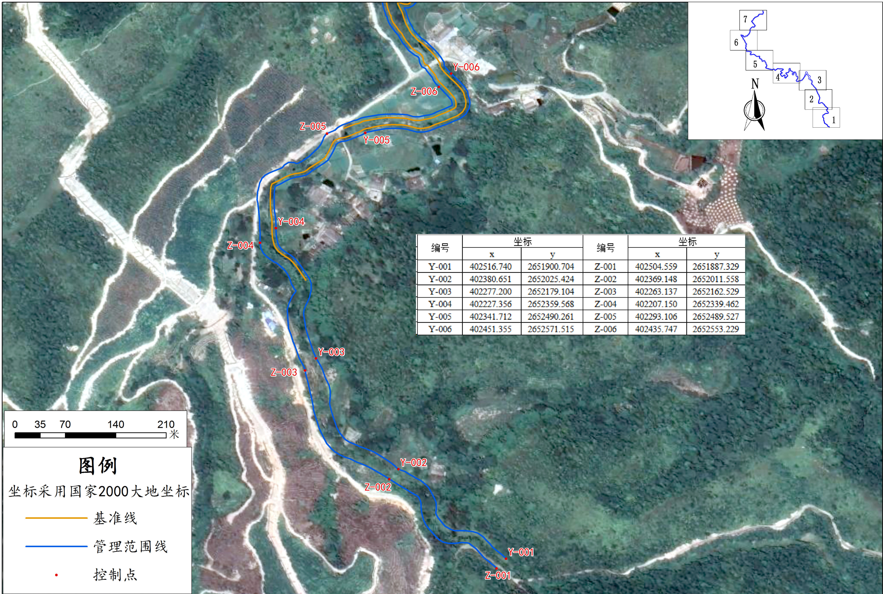
成江水支流赤双水河道管理范围线成果图（1/7）
