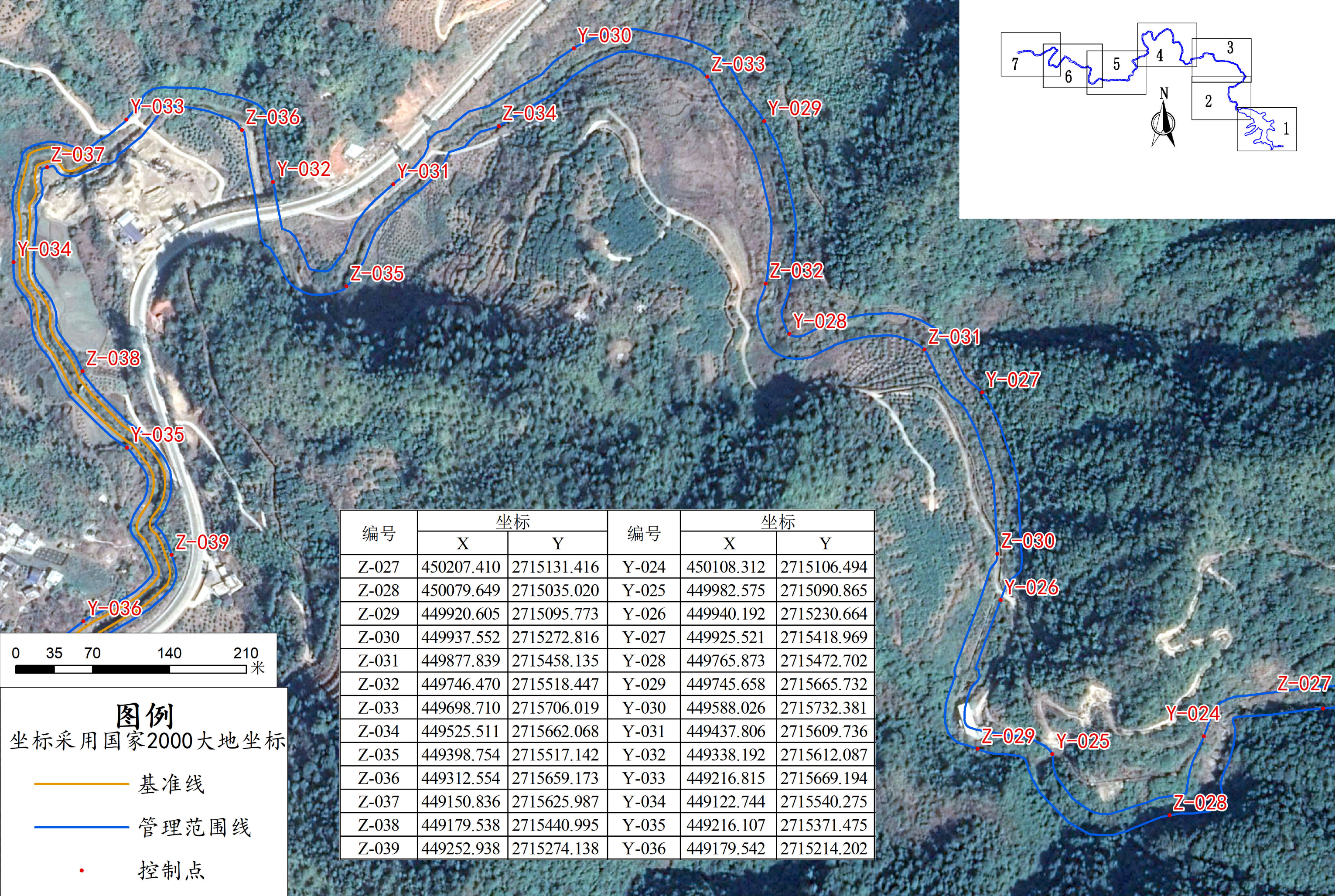
介溪水支流三塔水河道管理范围线成果图（4/7）
