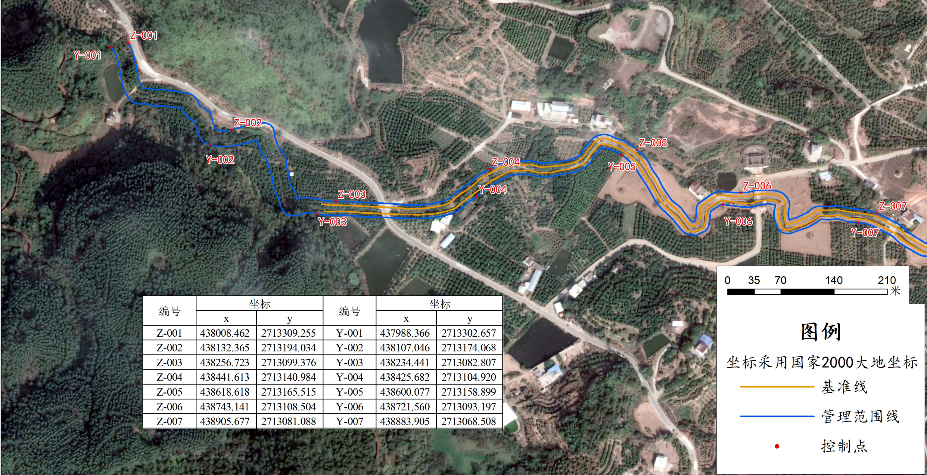
余坑水河道管理范围线成果图（1/3） 30
