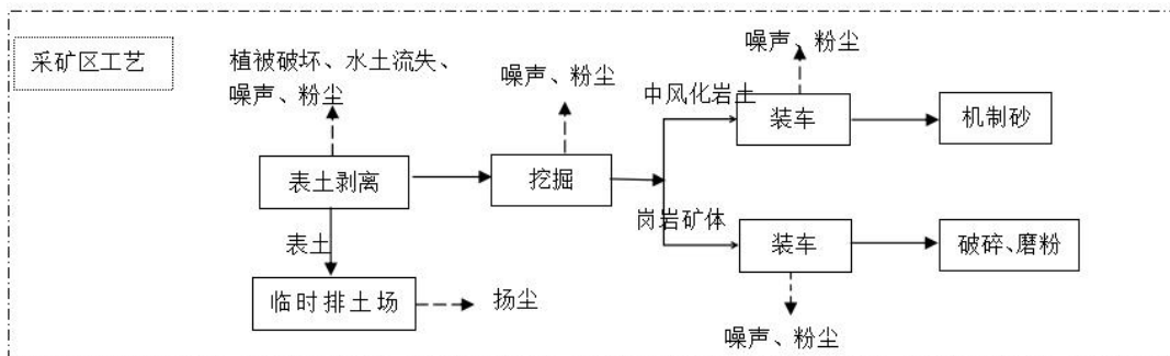
图 2-3 矿山开采工艺流程图
