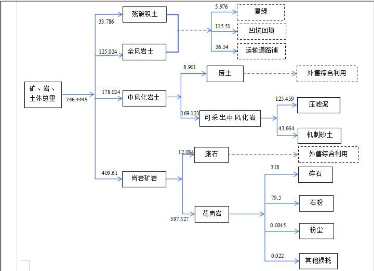
图 2-1 物料平衡图（单位：万 t/a）
