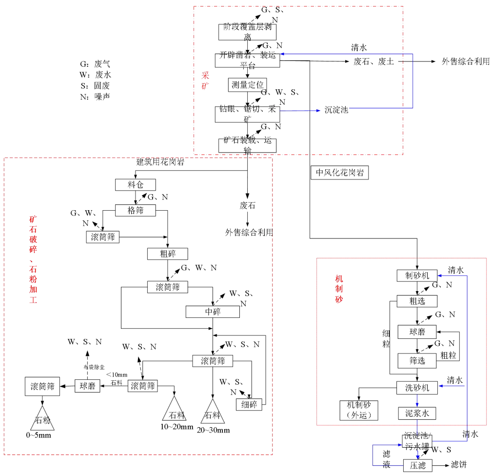
图 4-1 工艺流程及产物环节
