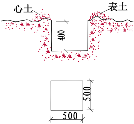
详图A 1:30
