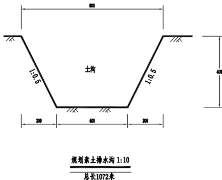
图 6-1 新修素土排水沟单体示意图
