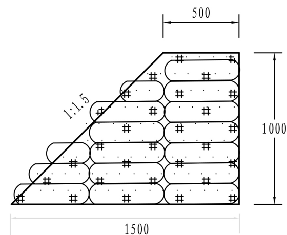
土方袋横断面图 1:20
