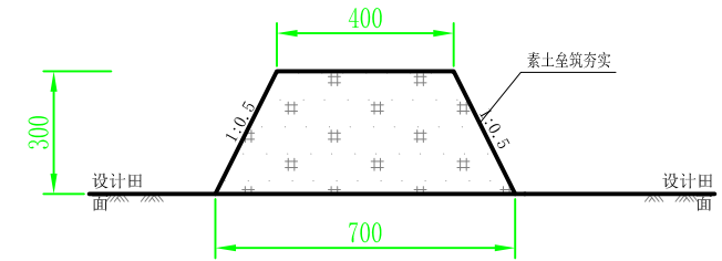
田埂横断面图 1:25
