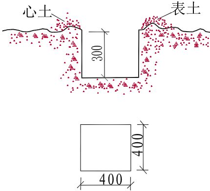
详图A 1:30
