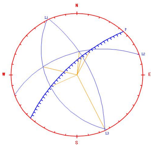
图 3-4 采场西面边坡 BP4 赤平投影图 图 3-5 采场北面边坡 BP1 赤平投影图
