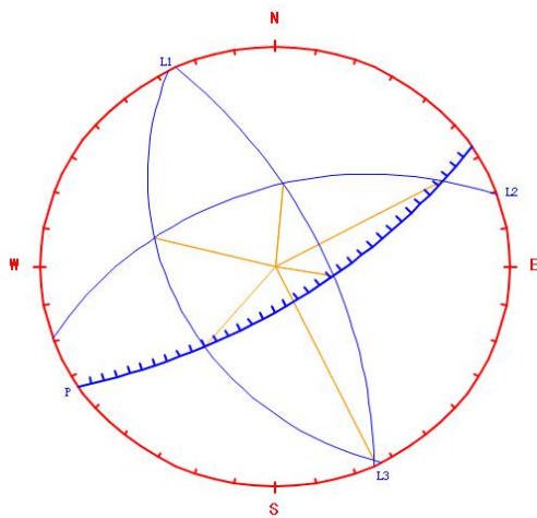
图 3-2 采场东面边坡 BP2 赤平投影图 图 3-3 采场南面边坡 BP3 赤平投影分析图
