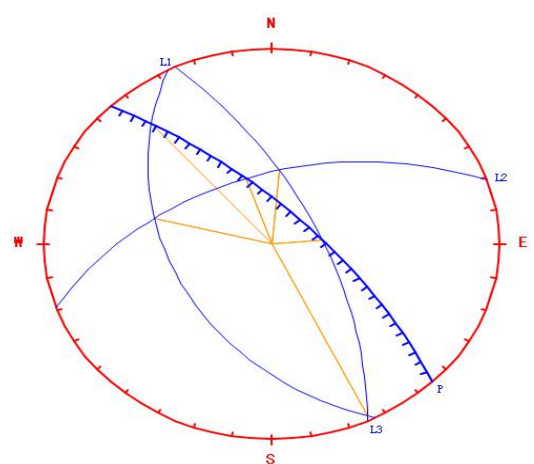
图 3-4 采场西面边坡 BP4 赤平投影图 图 3-5 采场北面边坡 BP1 赤平投影图
