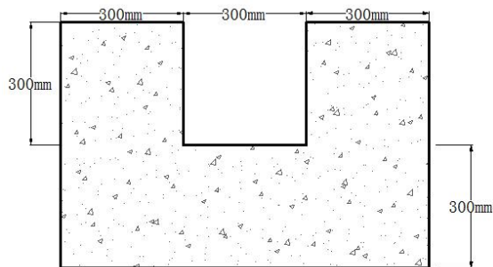
图 5-2 矿山道路截水沟断面示意图
