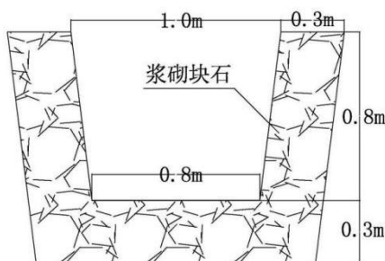
图 5-1 采场截排水沟断面示意图
