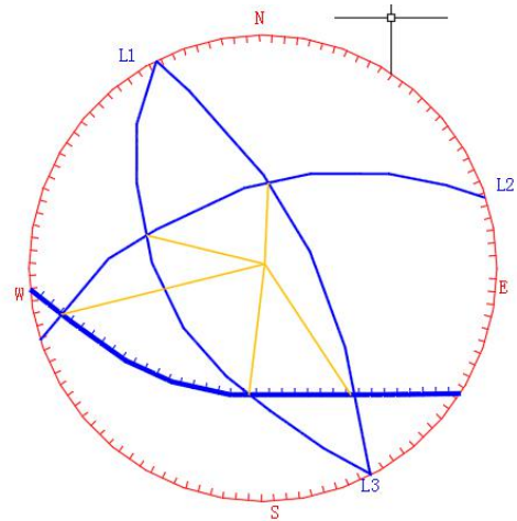
图 3-2 采场东面边坡 BP2 赤平投影图 图 3-3 采场南面边坡 BP3 赤平投影分析图
