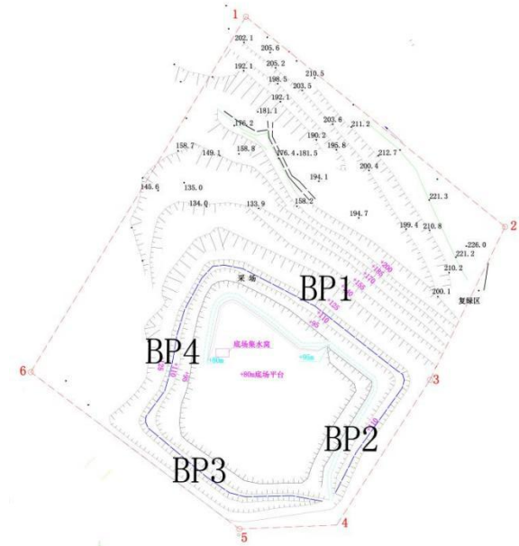
图3-1 矿山终了边坡类型示意图
