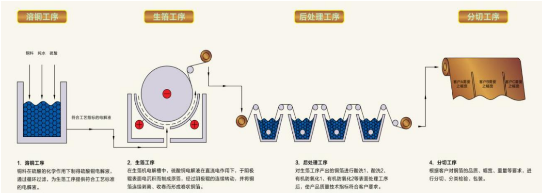
图 2-9 锂电铜箔制造主要工艺流程图
