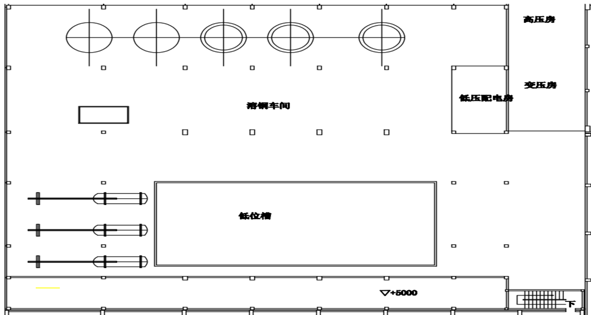
附图 5c 项目生产厂房溶铜车间平面布置图
