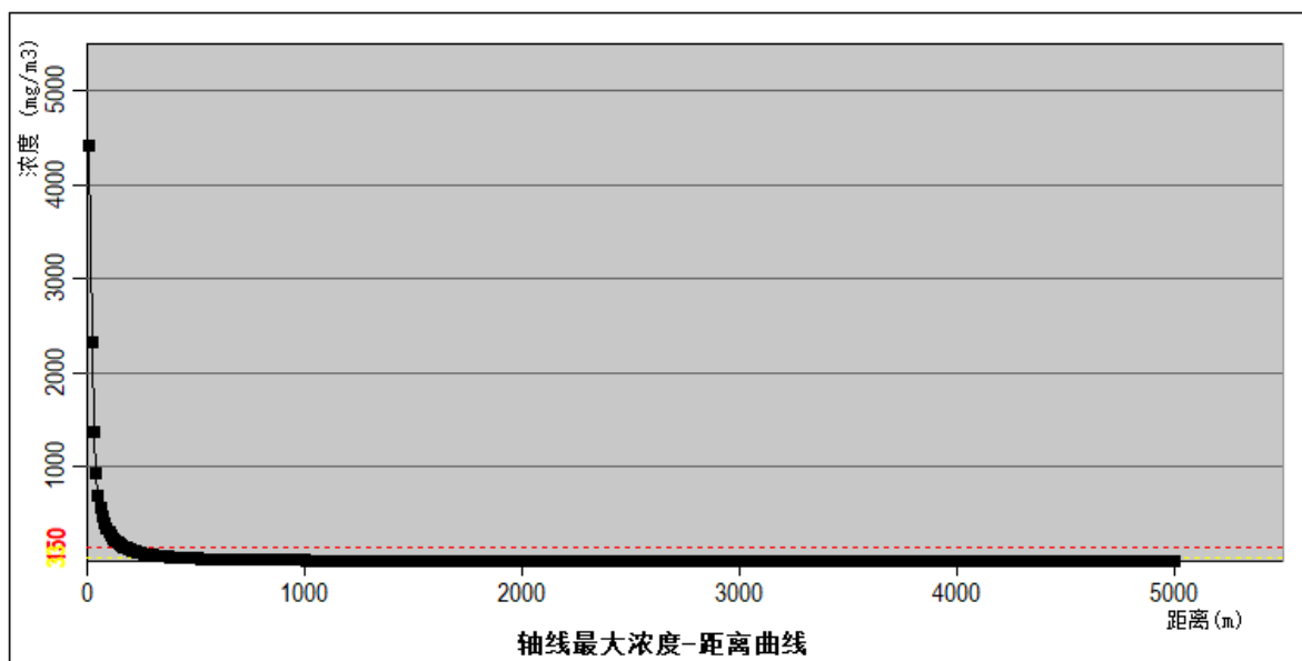
图 8.4-3 盐酸浓度随距离的变化曲线图
