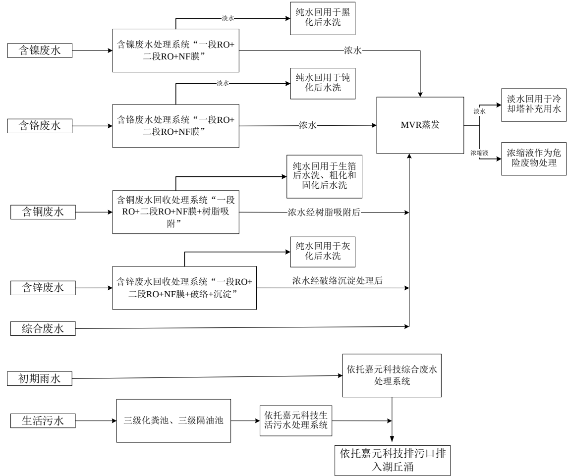
图 2-12 现有项目废水处理走向图
