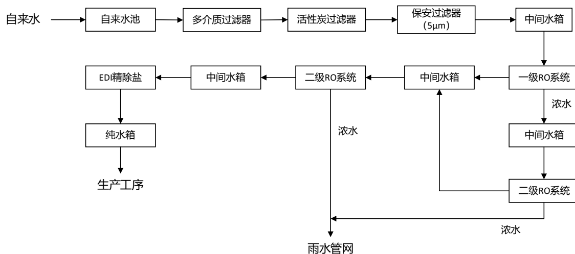
图 2-1 自来水制纯水系统工艺流程示意图
