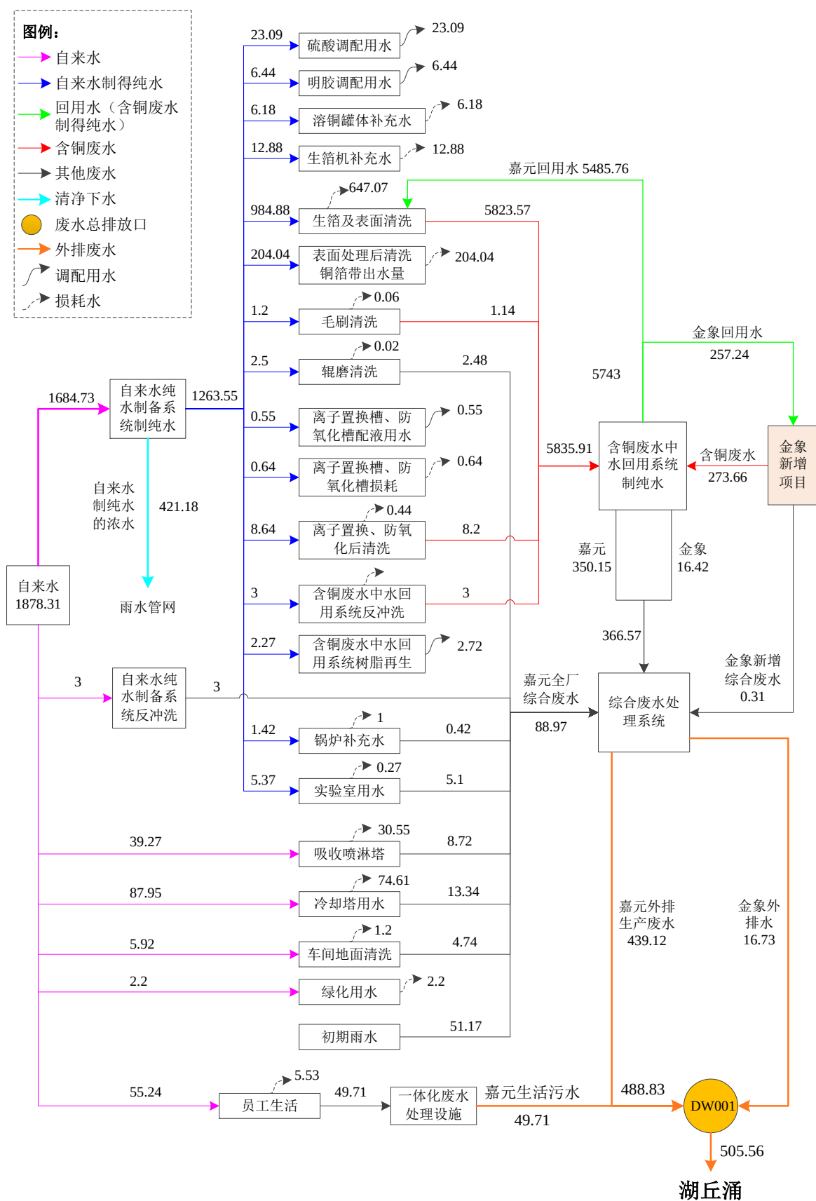
图 3.1-2 嘉元科技全厂及本扩建项目水平衡图 (单位: m³/d)
