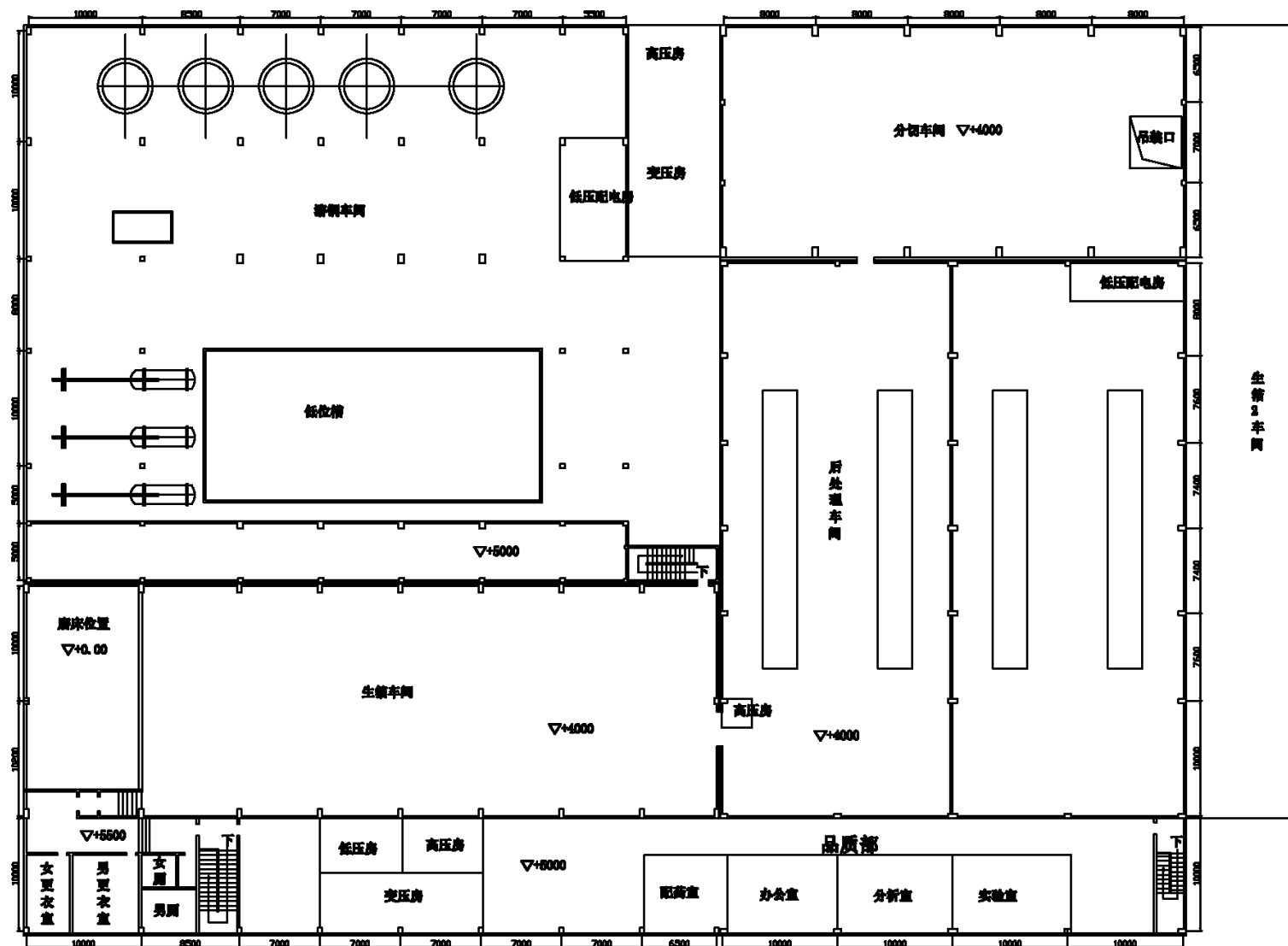
附图 5a 项目生产厂房一层平面布置图
