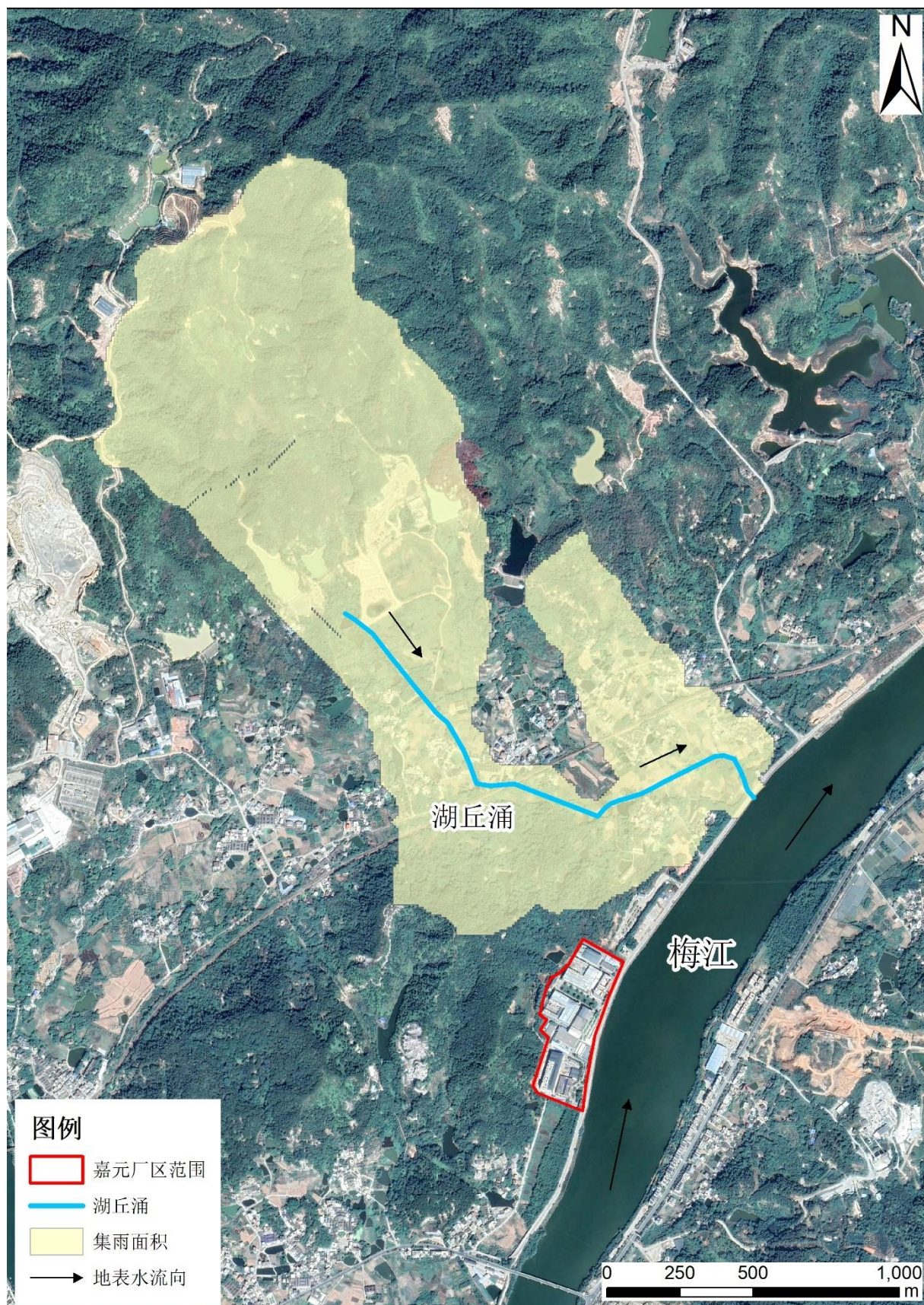
图 5.3-1 湖丘涌集雨范围示意图
