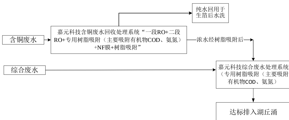
图 2-2 废水处理走向图
