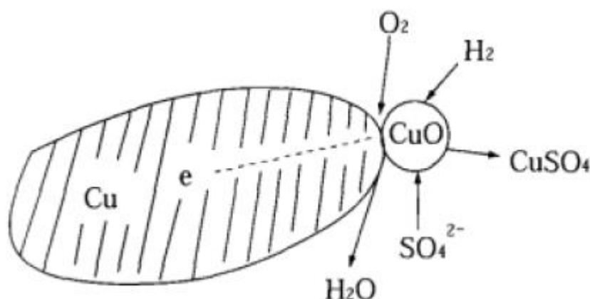
图 2-6 溶铜反应示意图
