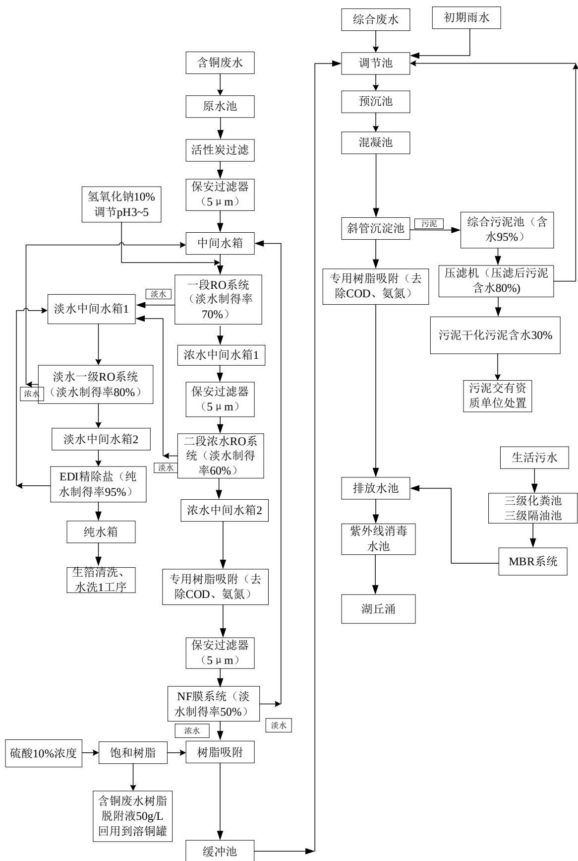
图 7.2-1 嘉元科技含铜废水、综合废水、生活污水处理工艺流程示意图
