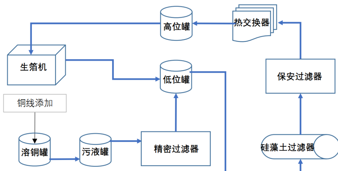
图 2-7 溶铜时硫酸铜溶液流向示意图
