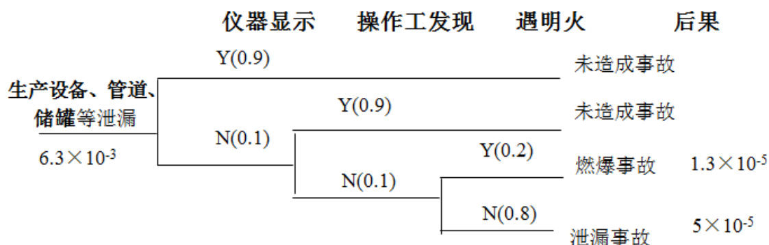
图 6.3-1 生产以及储罐系统事件树示意图
