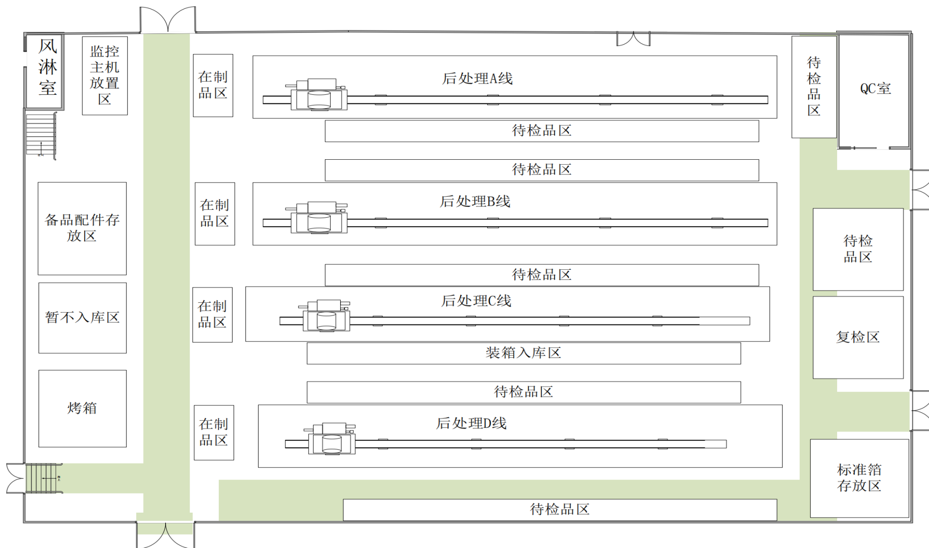
附图 5e 现有项目后处理车间平面布置图
