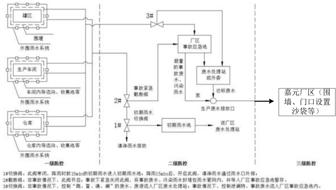
图 9.1-4 环境风险“三级防控”图
