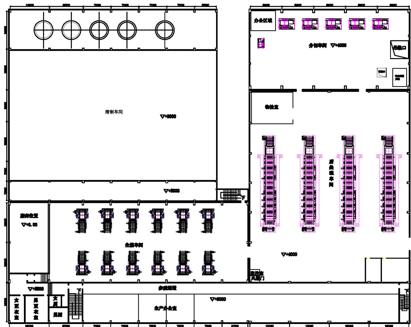
附图 5b 项目生产厂房二层平面布置图
