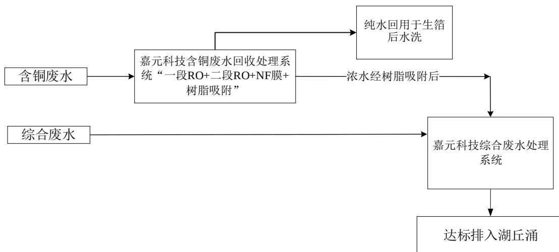
图 4-1 废水处理走向图
