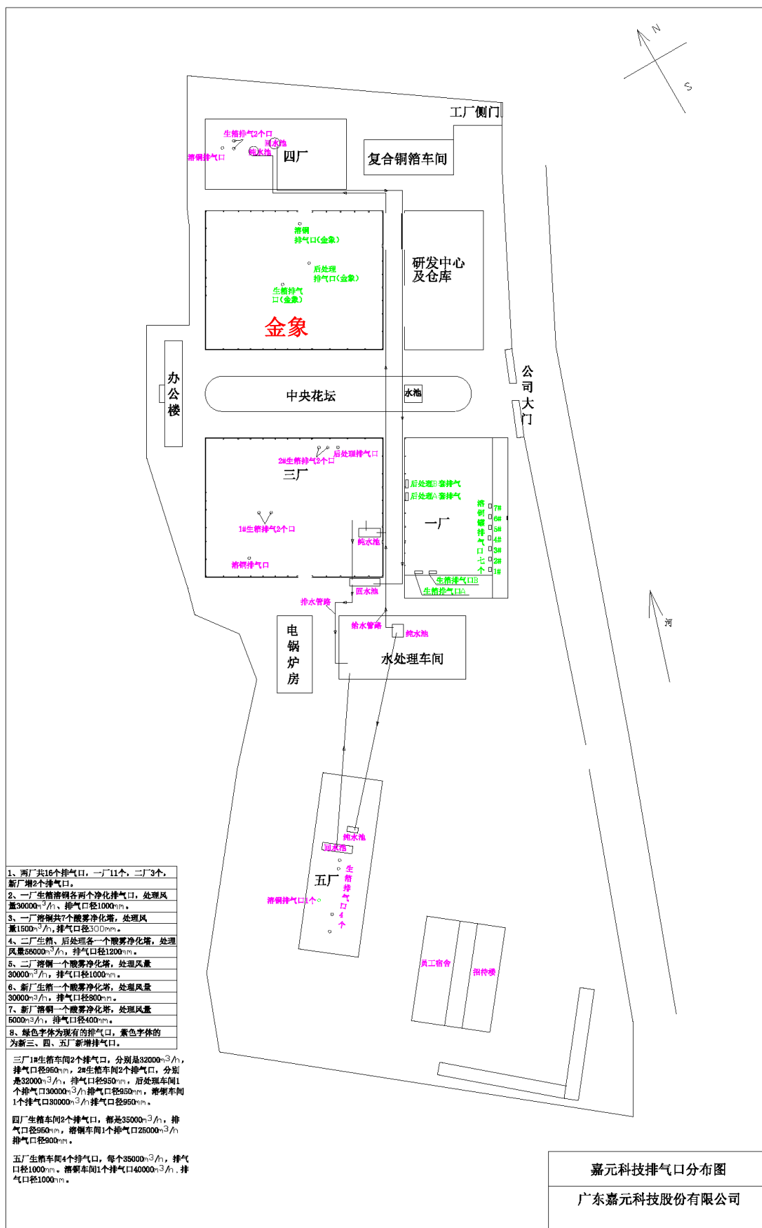
附图3 项目排气筒分布图
