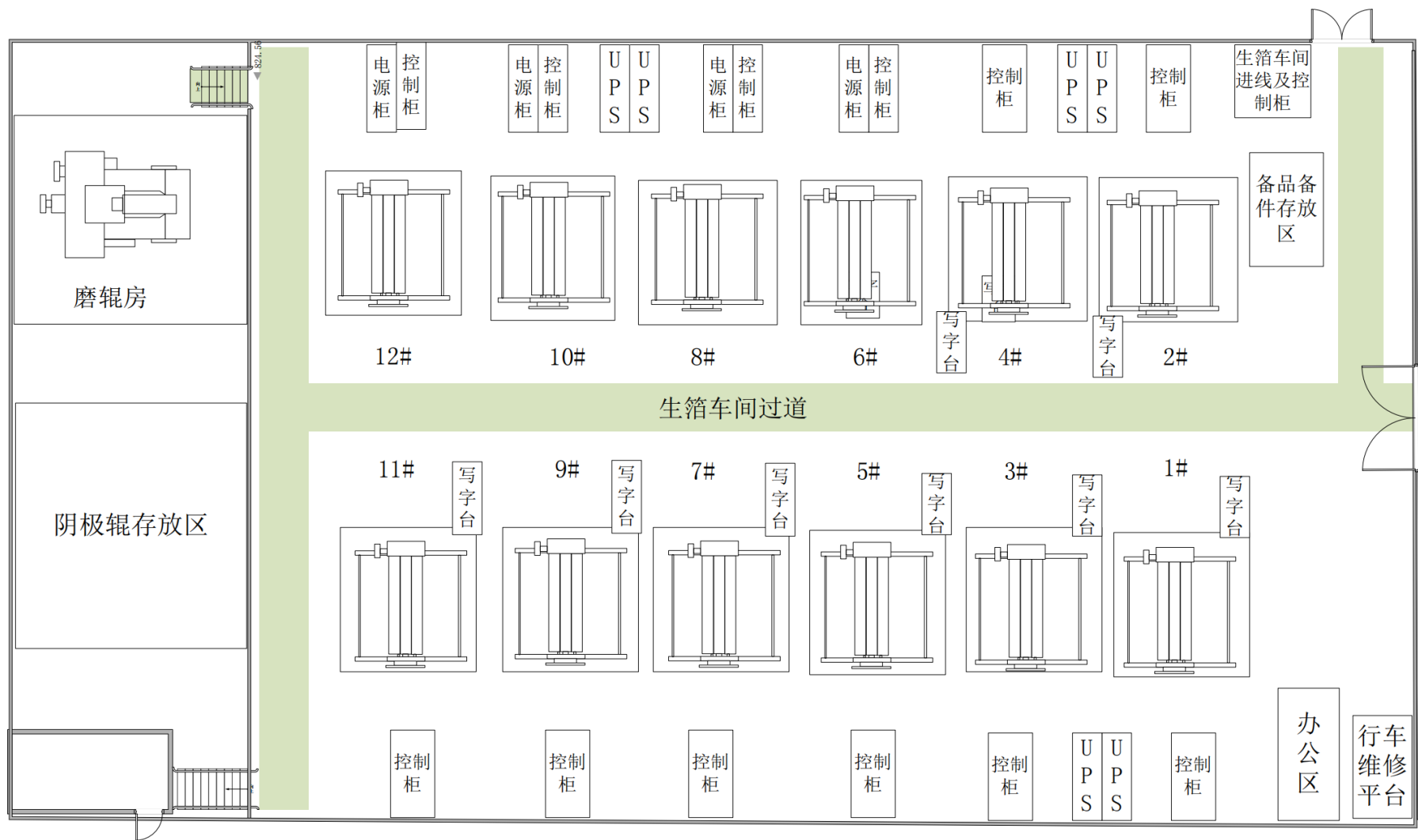
附图 5d 项目生箔车间平面布置图
