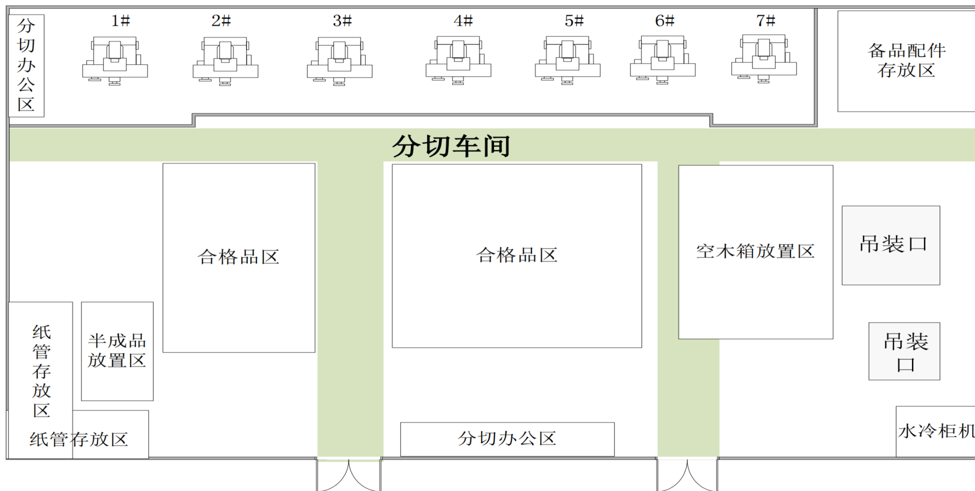
附图 5f 项目分切车间平面布置图
