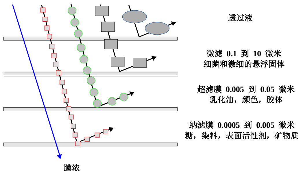
图 7.3-2 膜分离过程分类
