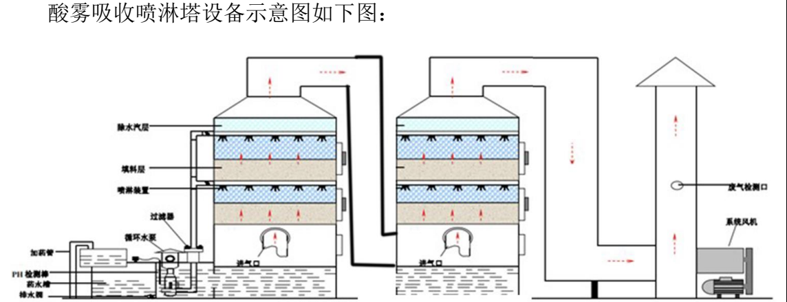
图 4-4 酸雾吸收喷淋塔设备示意图
