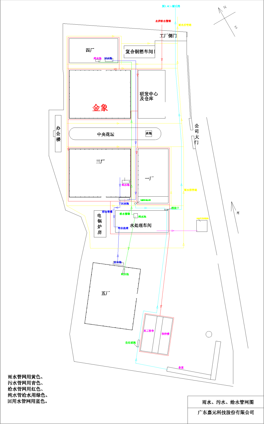
附图 4 项目雨污管网图
